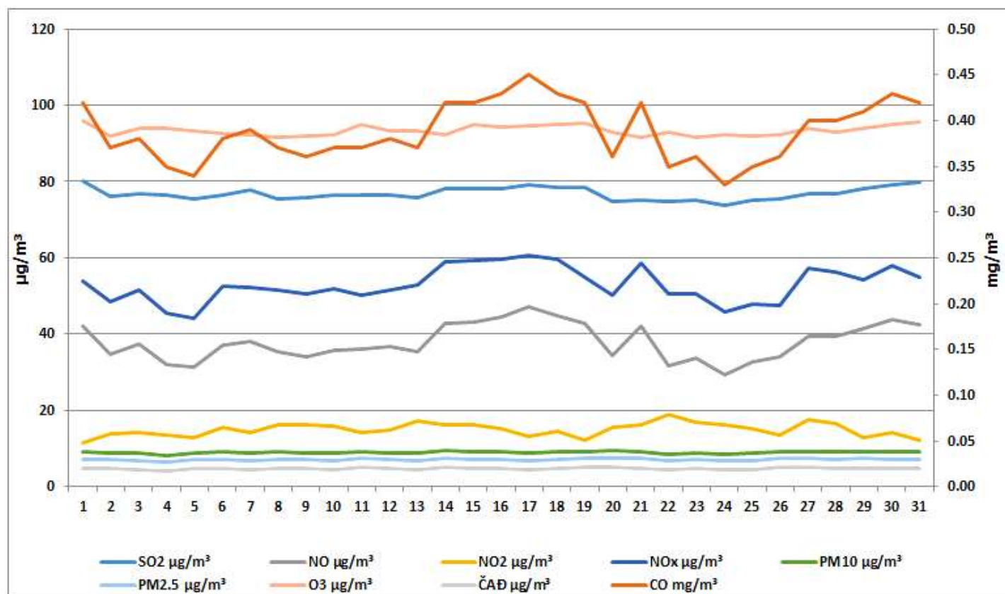
Дијаграм 6. Графички приказ просјечних имисијских дневних SO 2 , CO, NO, NO 2 , NO x , O 3 , ČАД, PM 2.5 и PM 10 за јул 2026. у Бијељини (мјерно мјесто Центар града)
