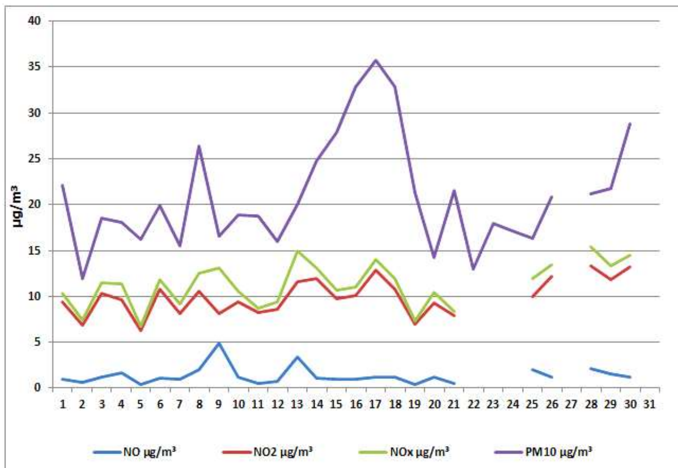
Дијаграм 11. Графички приказ просјечних имисијских дневних концентрација NO, NO 2 , NO x , PM 10 , O 3 и SO 2 за јул 2026. у Добоју (мјерно мјесто круг метеоролошке станице у Добоју)
