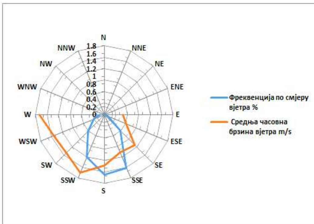
Слика 2. Приказ честине вјетра за јул 2026. у Гацку (мјерном мјесту круг ОШ „Свети Сава“).
