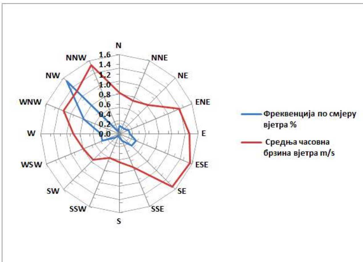
Слика 3. Приказ честине вјетра за јул 2026. године у Броду (мјерно мјесто Рафинерија нафте Брод а.д.)
