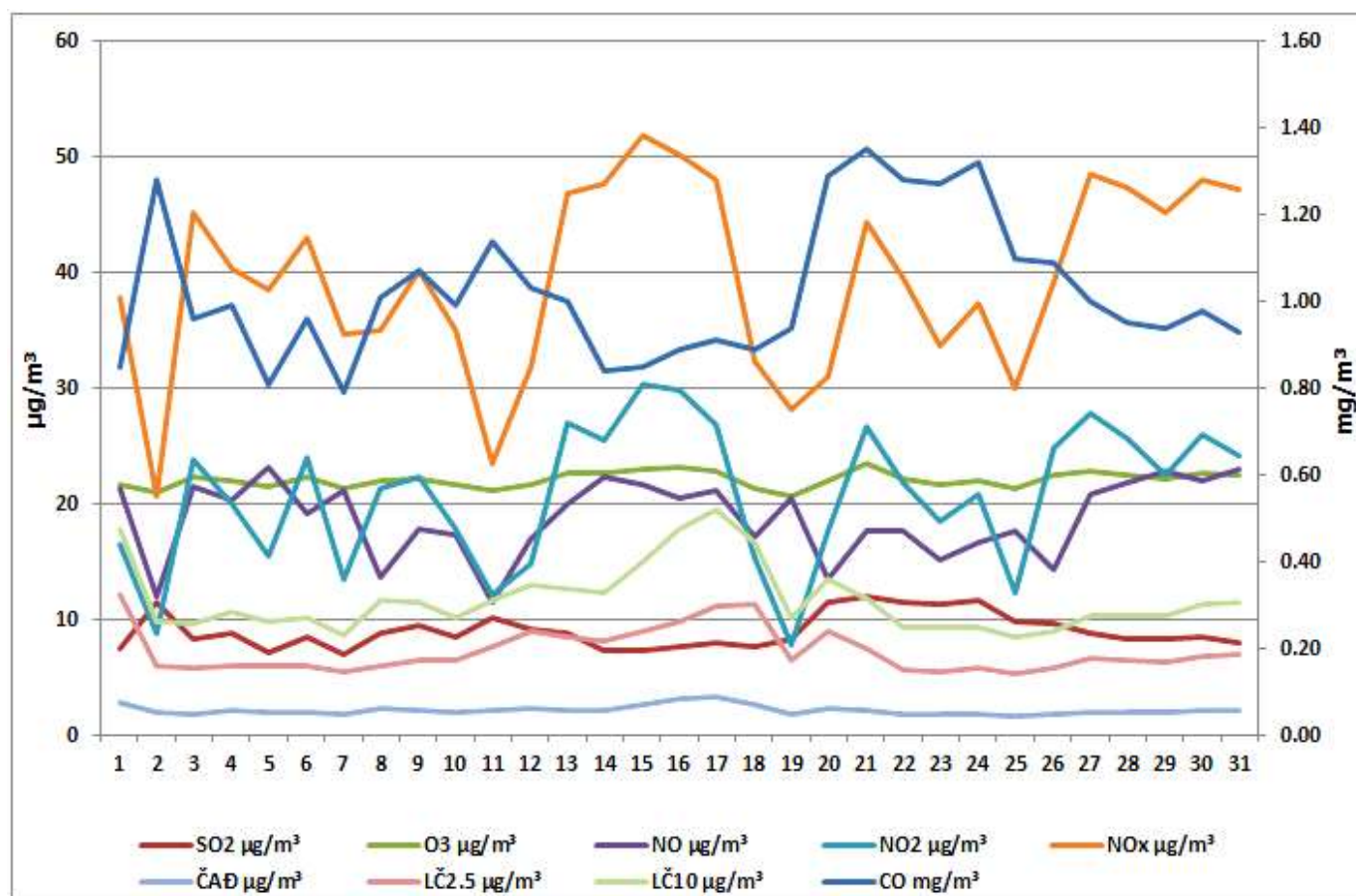
Дијаграм 3. Графички приказ просјечних имисијских дневних концентрација SO 2 , CO, NO, NO 2 , NO x , PM 2.5 , PM 10 , O 3 и ČАЂ за јул 2026. у Бањој Луци (мјерно мјесто Центар града).
