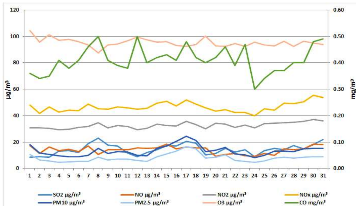
Дијаграм 12. Графички приказ просјечних имисијских дневних концентрација SO 2 , NO, NO 2 , NO x , O 3 , PM 10 , PM 2.5 и CO честица за јул 2026. у Градишци на мјерном мјесту „Културни центар“.
