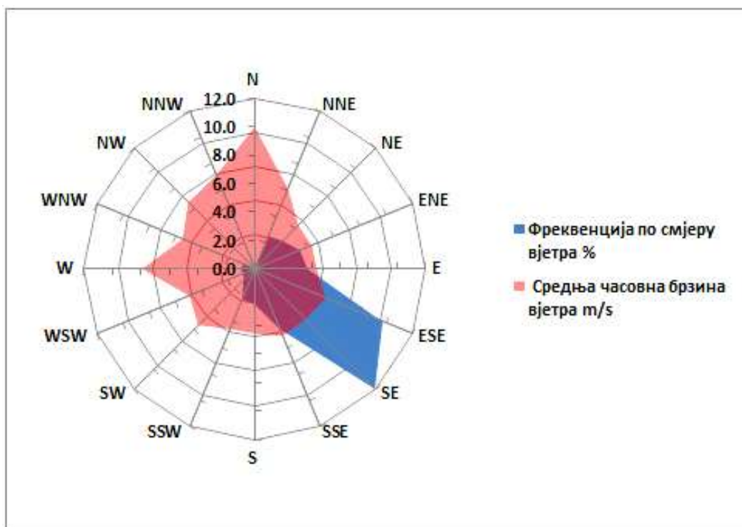
Слика 4. Приказ честине вјетра за јул 2026. године у Требињу (мјерно мјесто круг метеоролошке станице у Требињу)
