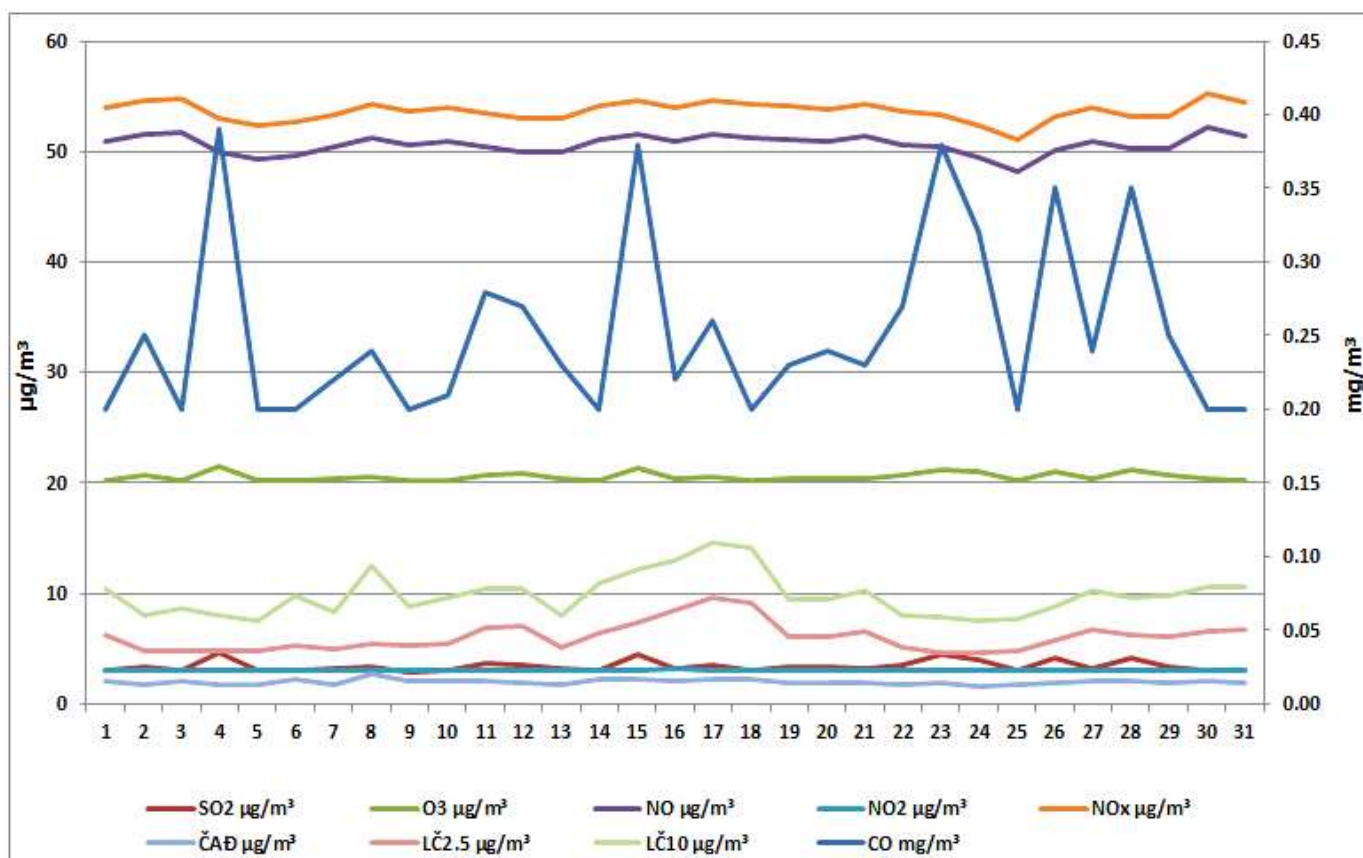
Дијаграм 4. Графички приказ просјечних имисијских дневних концентрација SO 2 , CO, NO, NO 2 , NO x , O 3 , PM 2.5 , PM 10 и ЧАД за јул 2026. у Бањој Луци (мјерно мјесто Борик).
