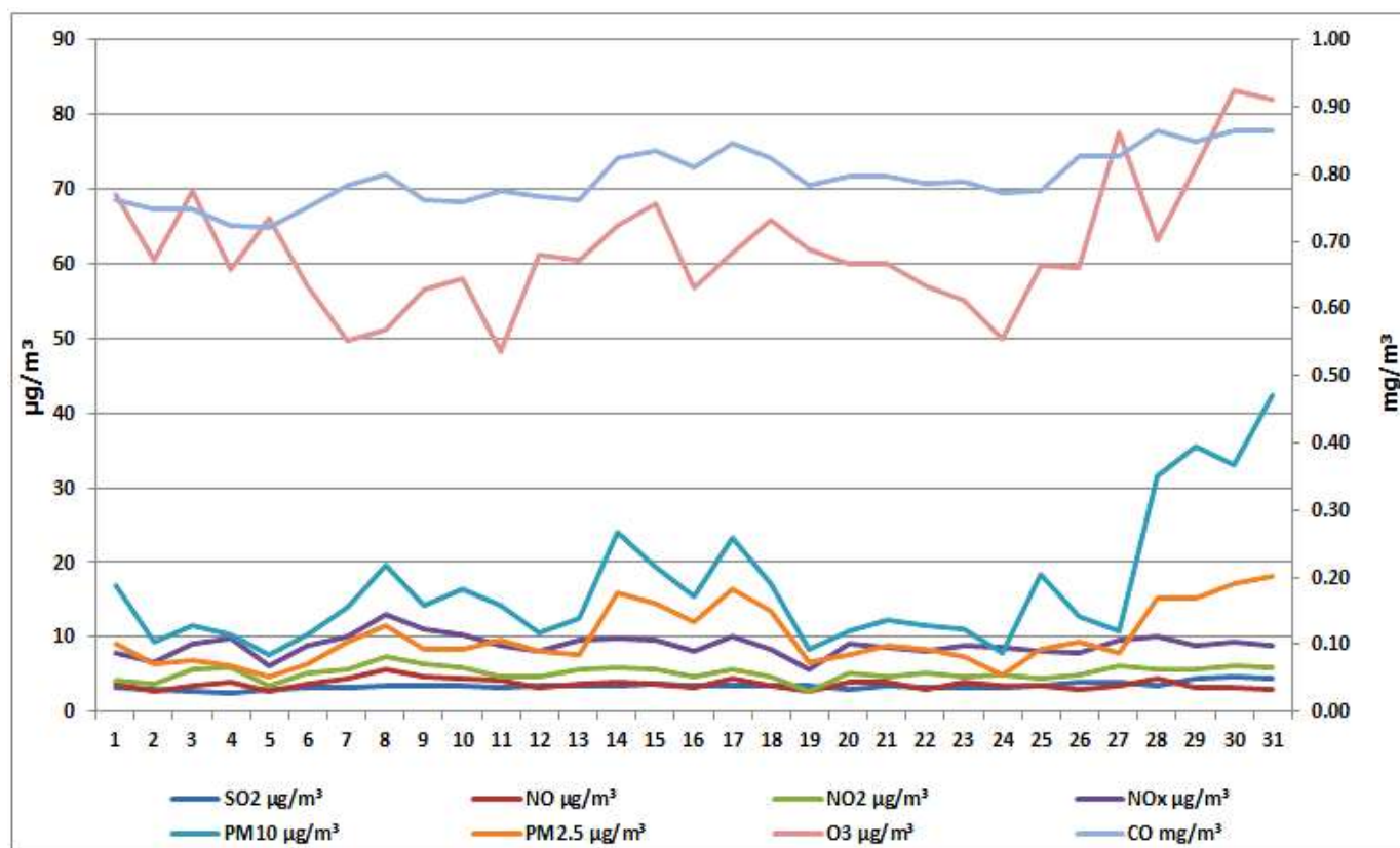
Дијаграм 5. Графички приказ просјечних имисијских дневних концентрација SO 2 , NO, NO 2 , NO x , PM 2.5 , PM 10 , CO и O 3 за јул 2026. у Приједору (мјерно мјесто круг метеоролошке станице у Приједору)
