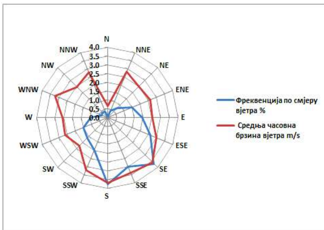
Слика 1. Приказ честине вјетра за јул 2026. У Бања Луци (мјерно мјесто Лазарево).
