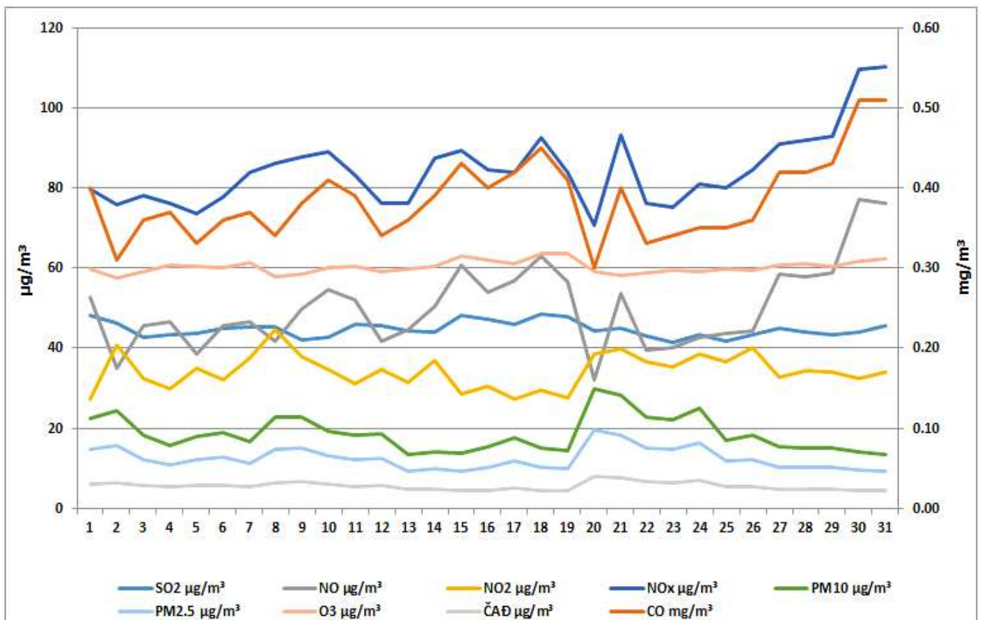
Дијаграм 7. Графички приказ просјечних имисијских дневних SO 2 , CO, NO, NO 2 , NO x , O 3 , ЧАД, PM 2.5 и PM 10 за јул 2026. у Бијељини (мјерно мјесто Топлана).
