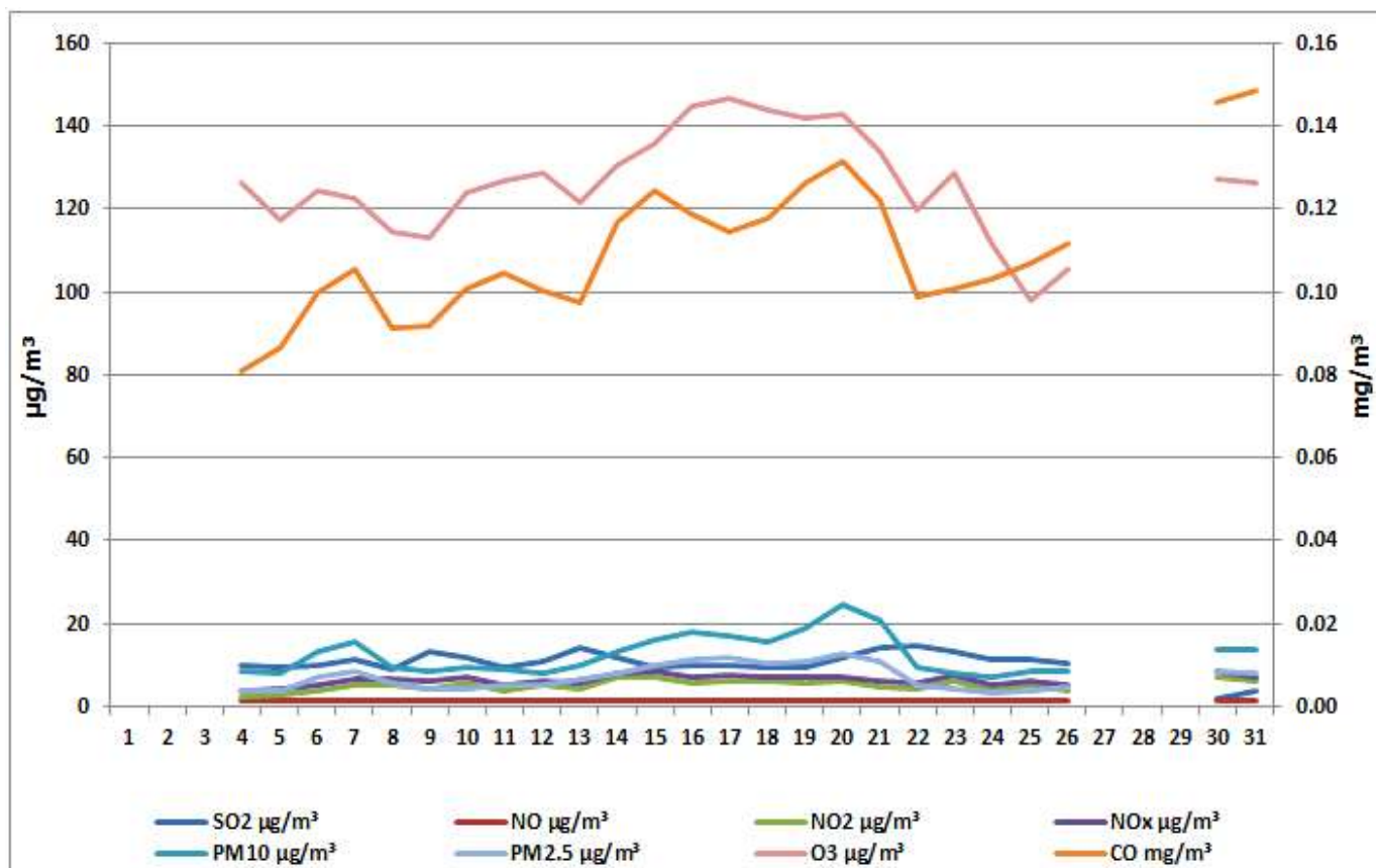
Дијаграм 10. Графички приказ просјечних имисијских дневних концентрација SO 2 , NO, NO 2 , NO x , CO, PM 10 , O 3 и PM 2.5 честица за јул 2026. у Требињу (мјерно мјесто круг метеоролошке станице у Требињу)
