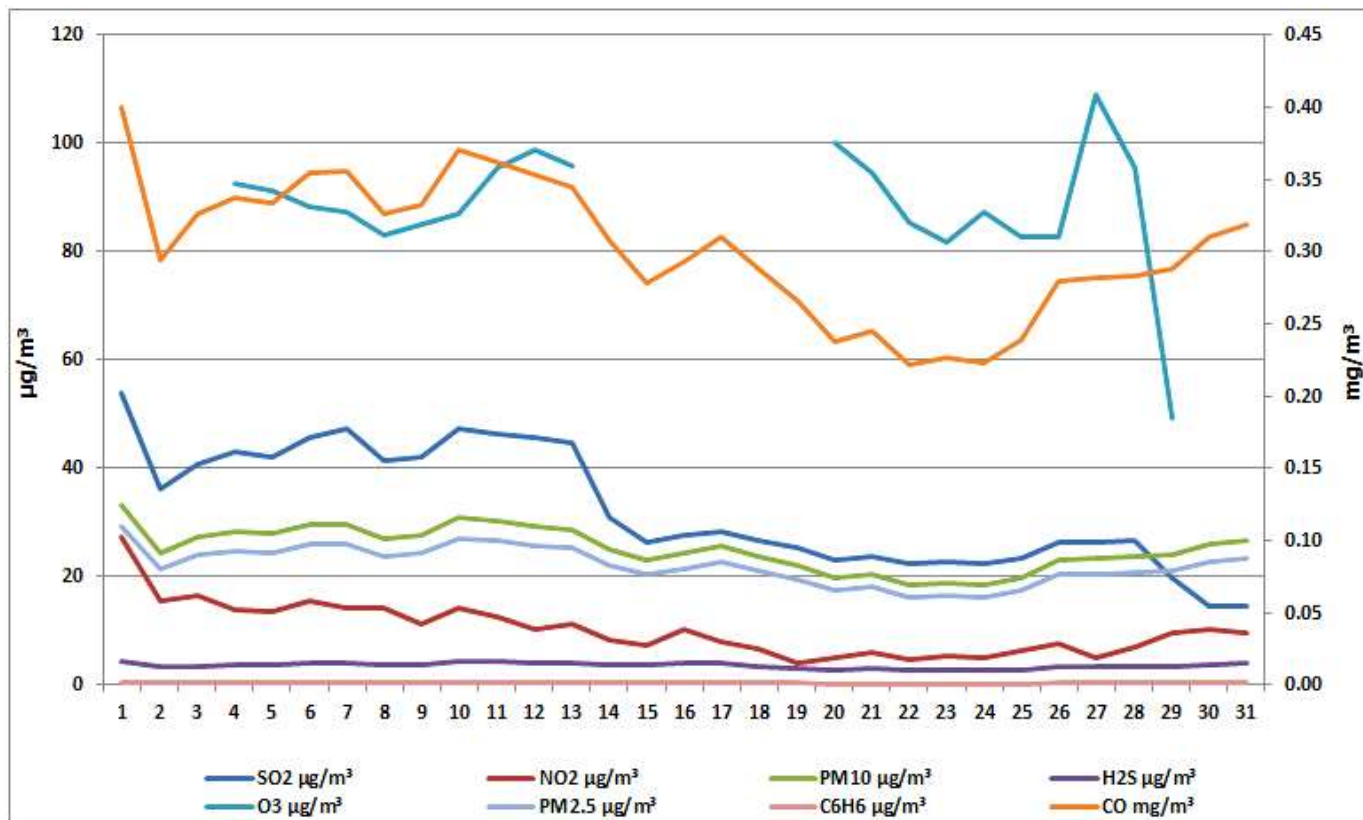
Дијаграм 9. Графички приказ просјечних имисијских дневних концентрација SO 2 , CO, O 3 , C 6 H 6 , H 2 S, NO 2 , PM 2.5 , и PM 10 честица за јул 2026. у Броду (мјерно мјесто Рафинерија нафте Брод а.д.)
