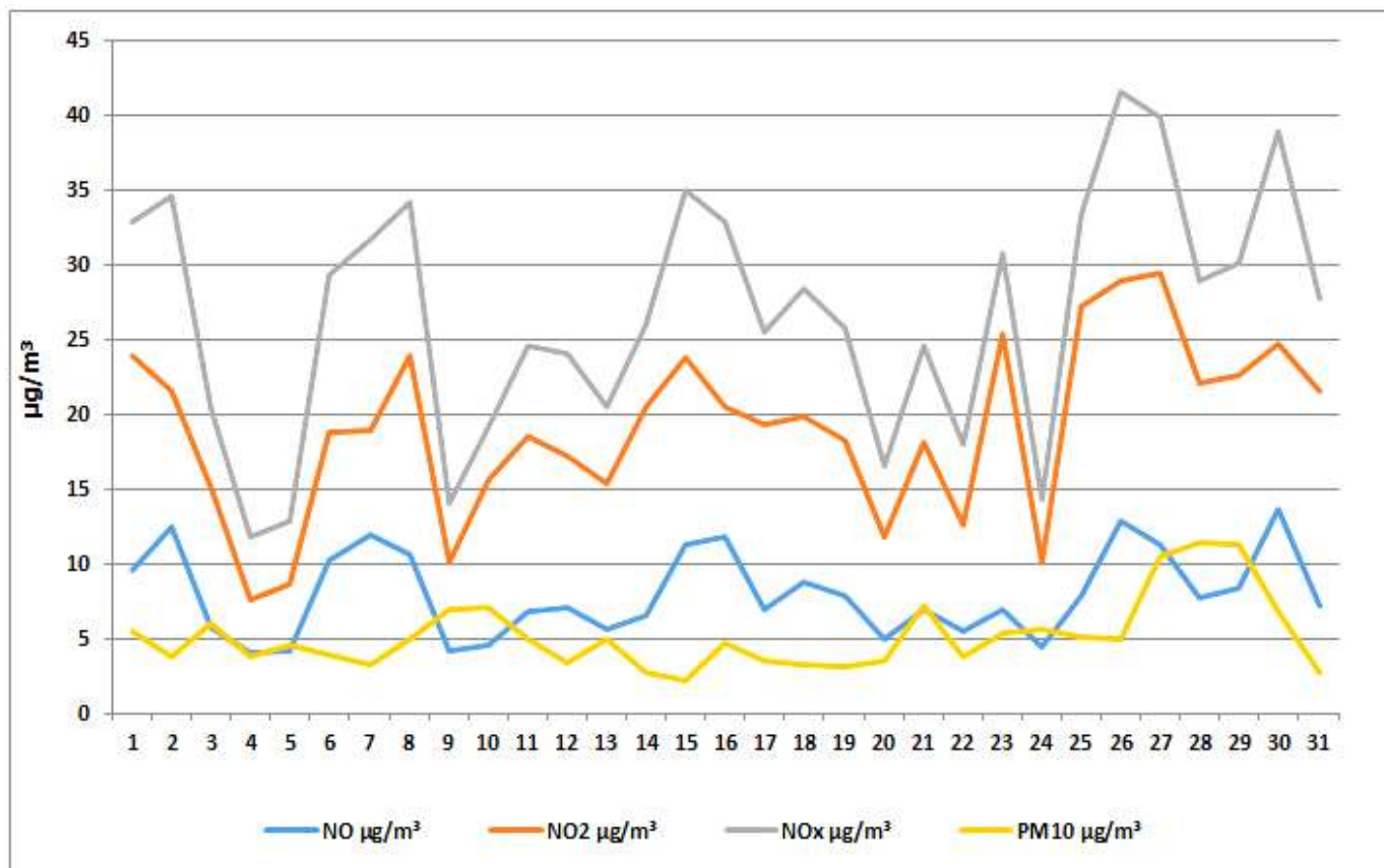
Дијаграм 8. Графички приказ просјечних имисијских дневних концентрација PM_{10} , NO, NO_2 и NO_x за јул 2026. у Гацку (мјерном мјесту круг ОШ „Свети Сава“).
