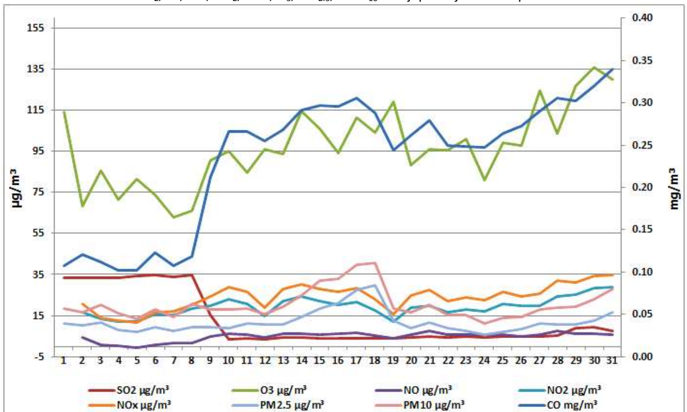
Дијаграм 1. Графички приказ просјечних имисијских дневних концентрација SO 2 , CO, NO, NO 2 , NO x , O 3 , PM 2.5 и PM 10 за јул 2026 у Бањој Луци (мјерно мјесто Лазарево).
